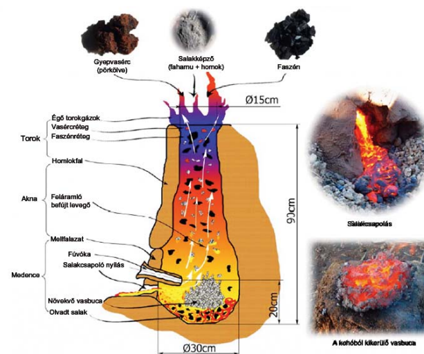
A bucafemence felépítése, betétanyagai, salakja és vascúdjája
