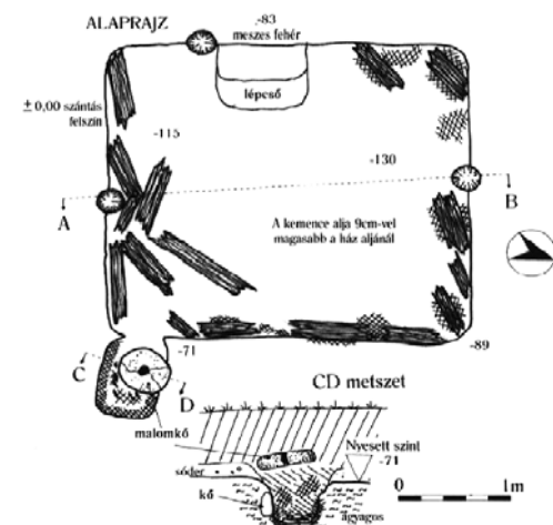
Fertőszentmiklós - 11. századi ház alaprajza és metszete. (A szerző ásatása)
